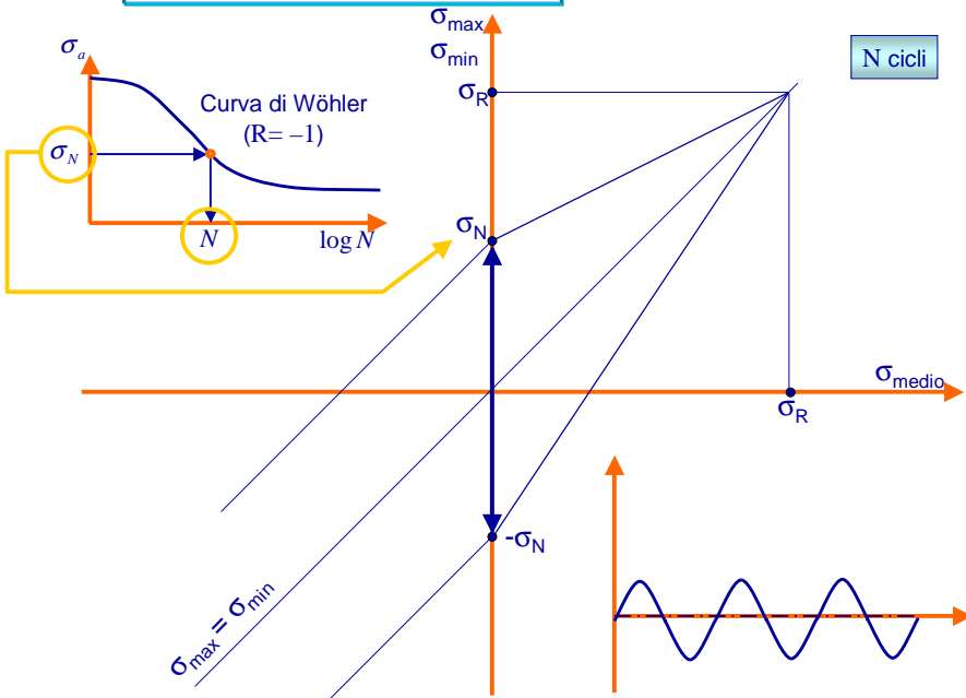
Diagramma di Goodman-Smith
